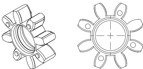
Fig. 18.34 Elastomer insert
